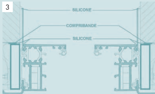
pose sur précadre
