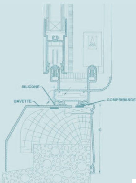
pose avec habillages extérieur et intérieur complets
