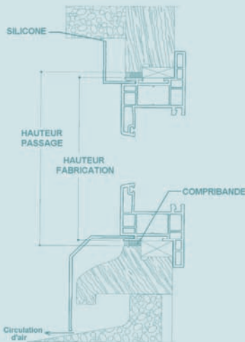
pose avec habillage extérieur complet et habillage intérieur partiel
