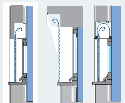
Pose tableau Enroulement dans un coffre bois intérieur
