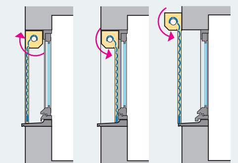
Pose tableau Enroulement intérieur
